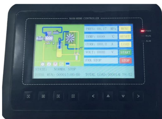
Рис. 1. Дисплей контроллера
